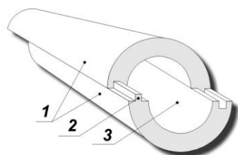
1 - скорлупы 2 - замковое соединение 3 - изолируемая поверхность
